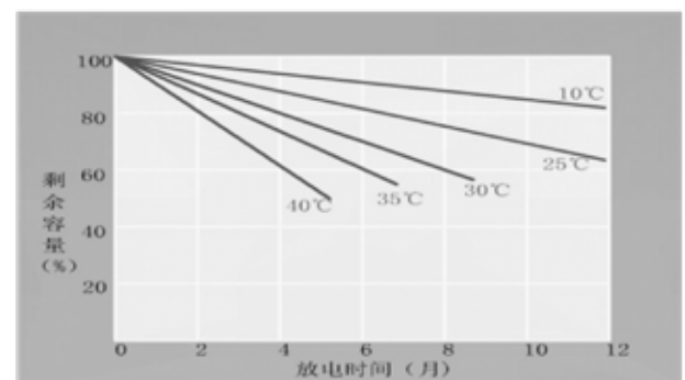
自放电特性
